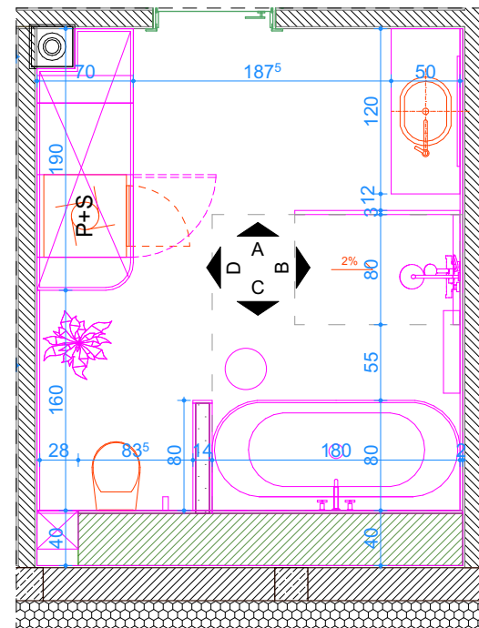
FRAGMENT RZUTU ŁAZIENKI GŁÓWNEJ NA GÓRZE
