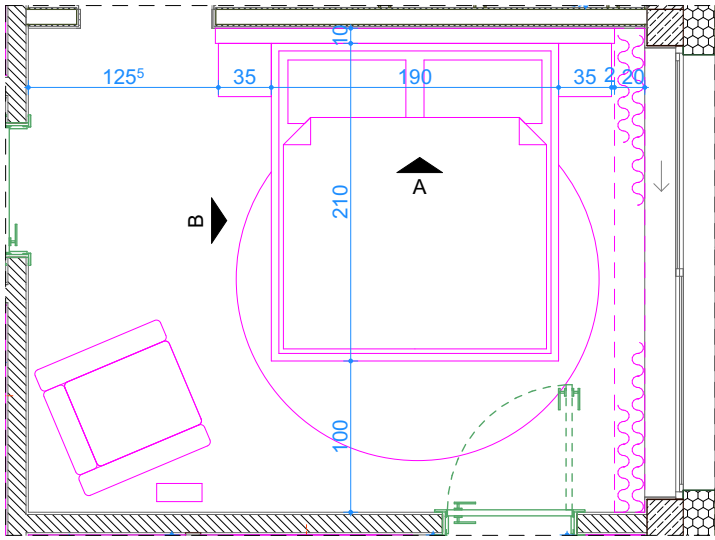
FRAGMENT RZUTU SYPIALNI MASTER
