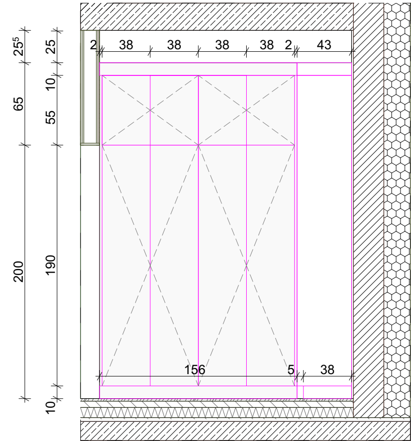
WIDOK A - FRONTY
