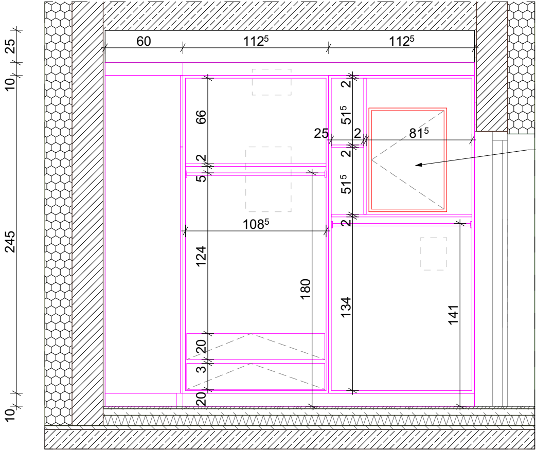
WIDOK B - WNĘTRZA
