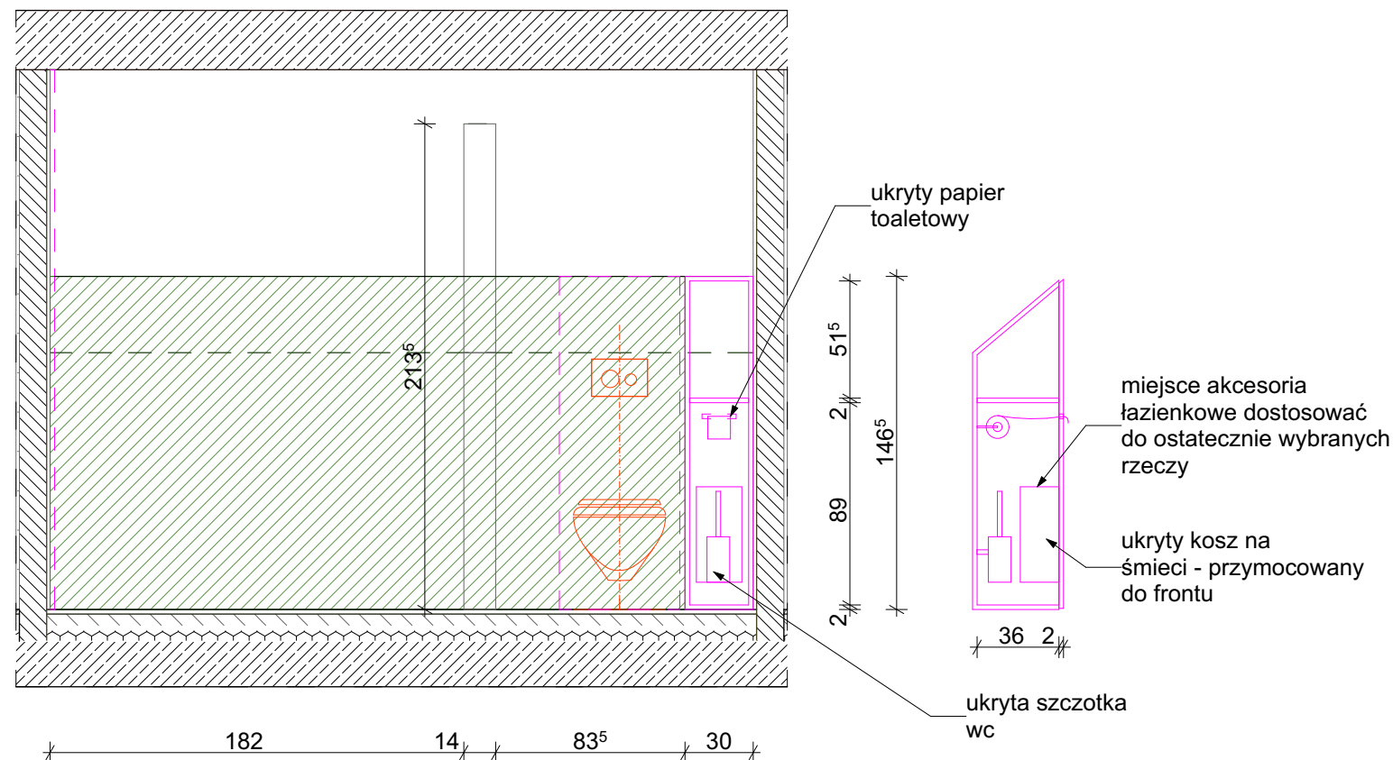
WIDOK C - WNĘTRZA
