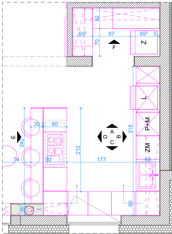
FRAGMENT RZUTU KUCHNI I SPIŻARNI
