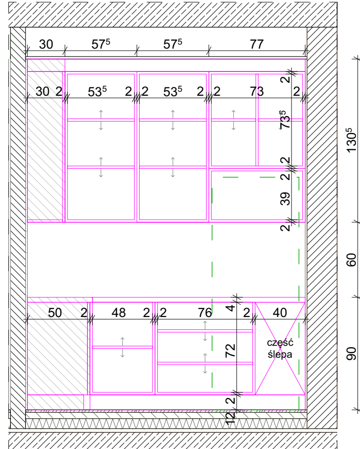
WIDOK F - WNĘTRZA
