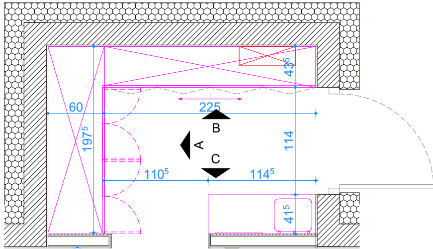
FRAGMENT RZUTU WIATROŁAPU
