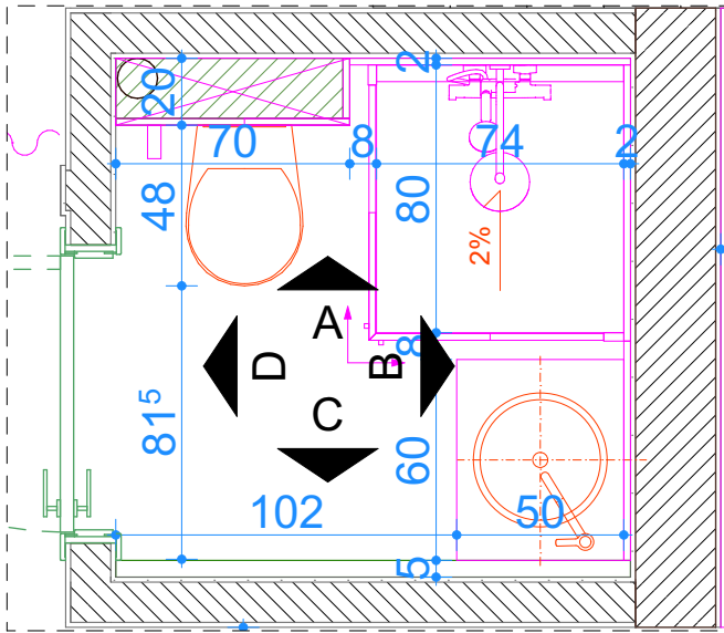
FRAGMENT RZUTU ŁAZIENKI NA DOLE
