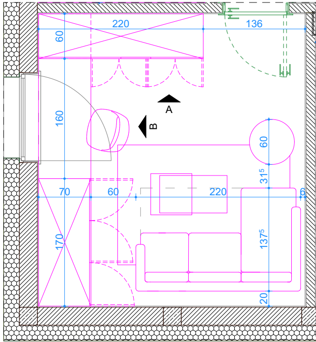
FRAGMENT RZUTU POKOJU GOŚCINNEGO
