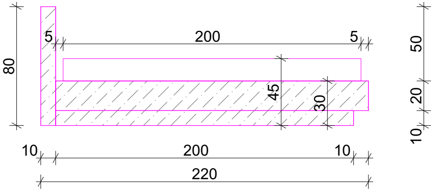
WIDOK Z BOKU NA ŁÓŻKO
