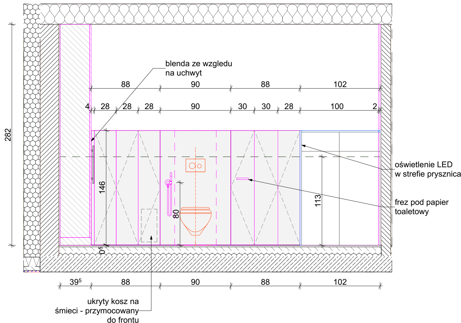
WIDOK C - FRONTY
