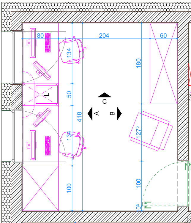
FRAGMENT RZUTU GABINETU
