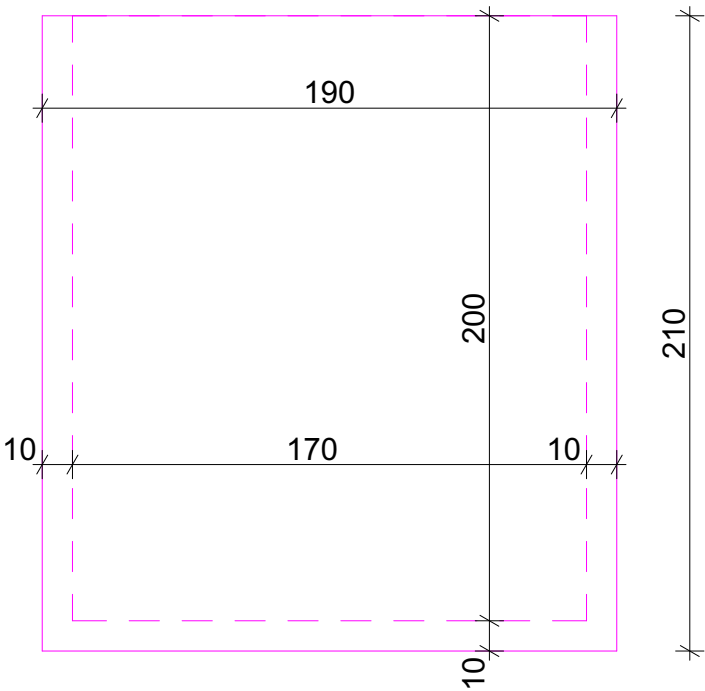
WIDOK Z GÓRY NA RAMĘ ŁÓŻKA
