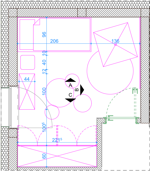
FRAGMENT RZUTU POKOJU ANTKA
