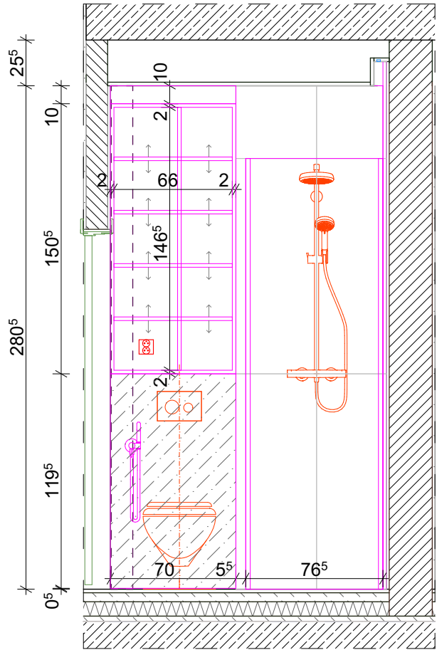
WIDOK A - WNĘTRZA
