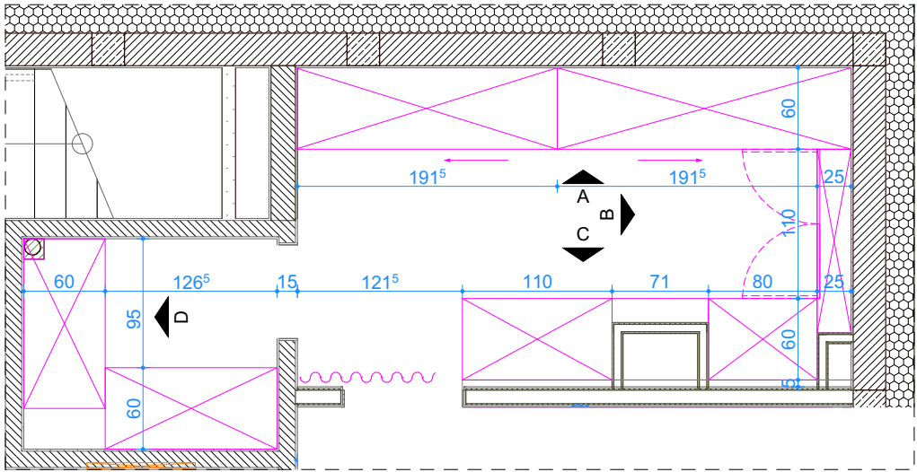
FRAGMENT RZUTU GARDEROBY
