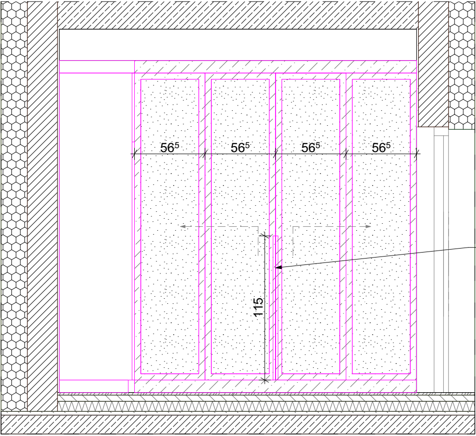
WIDOK B - FRONTY
