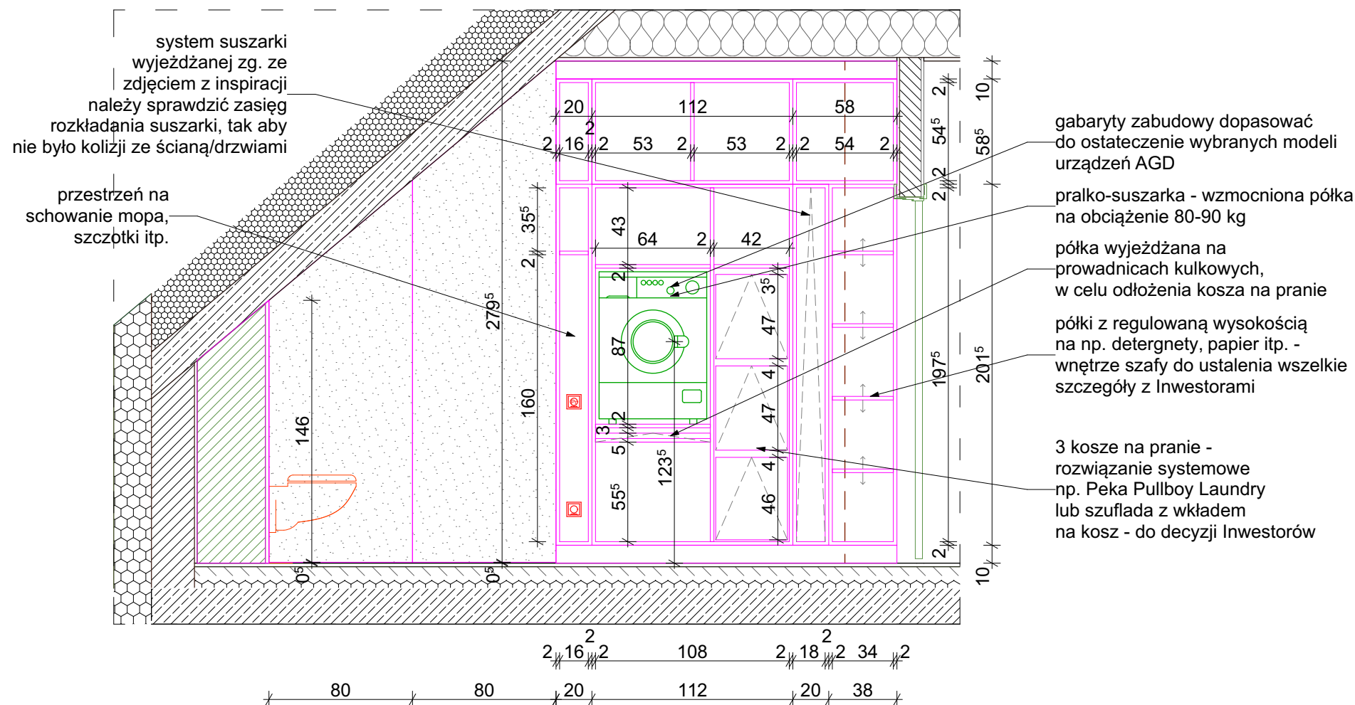
WIDOK D - WNĘTRZA
