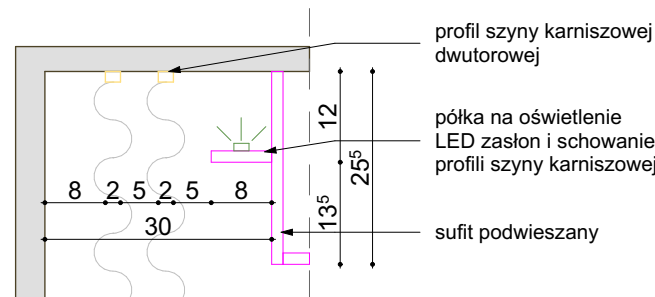
DETAL MONTAŻU SZYNY PODWÓJNEJ KARNISZOWEJ
