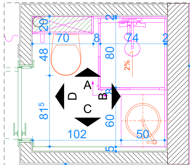
FRAGMENT RZUTU ŁAZIENKI NA DOLE
