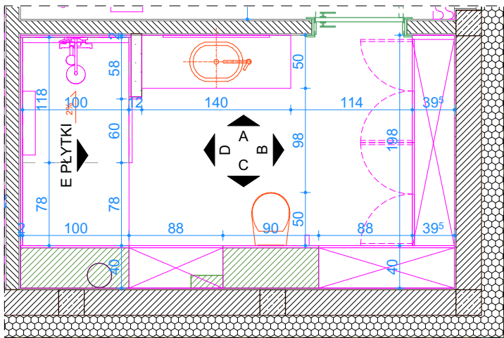
FRAGMENT RZUTU ŁAZIENKI PRZY SYPIALNI NA GÓRZE
