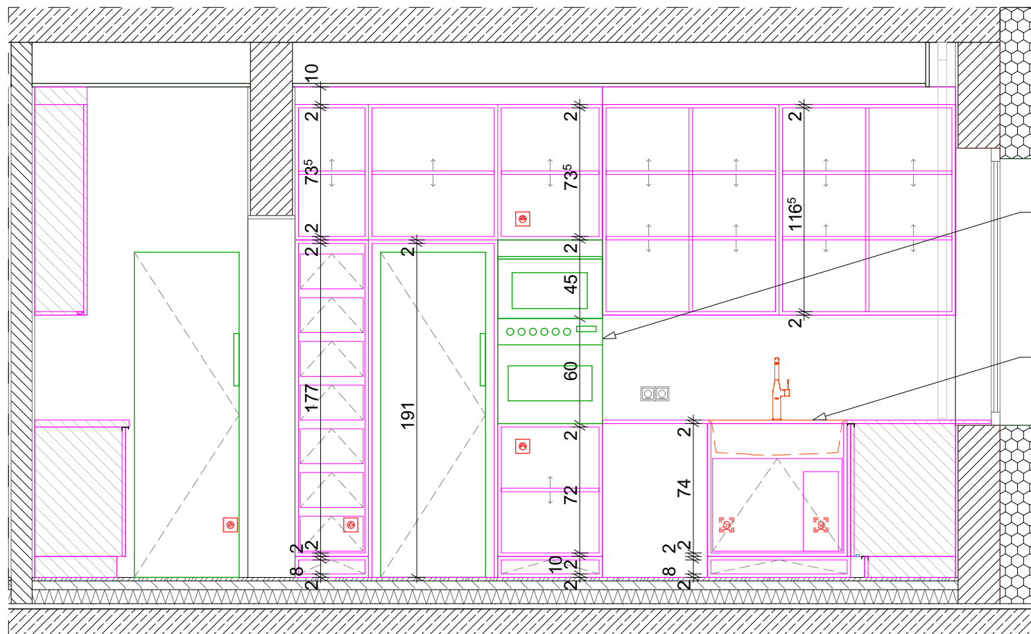
WIDOK B - WNĘTRZA
