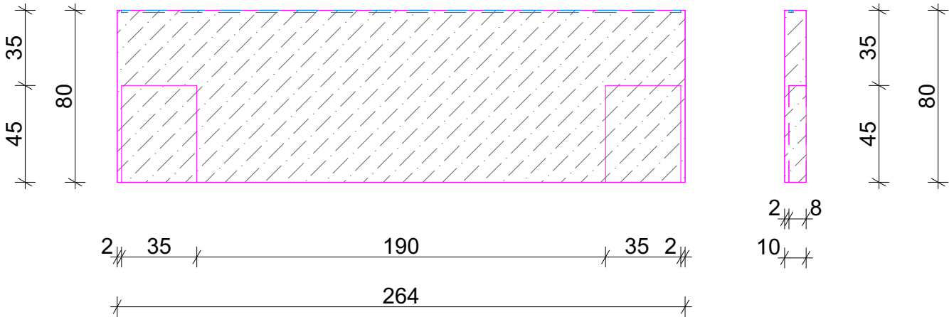
WIDOK FRONTALNY NA WEZGŁOWIE
