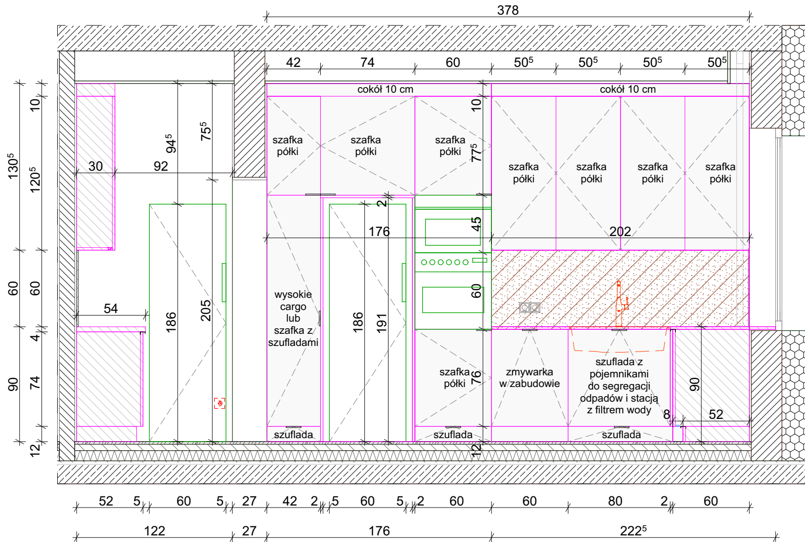
WIDOK B - FRONTY
